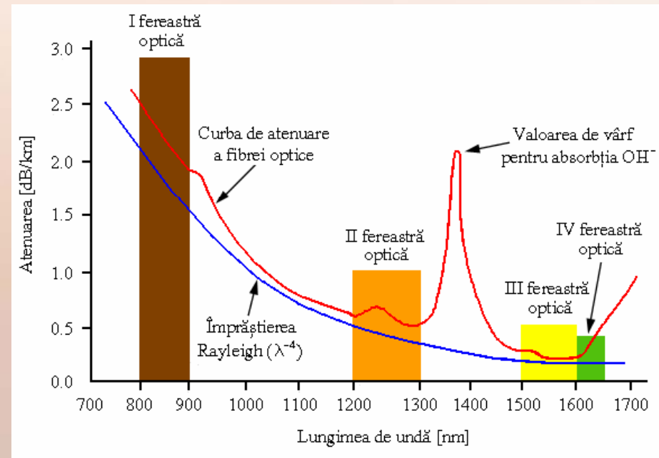
Atenuarea fibrei optice in functie de lungimea de unda.
